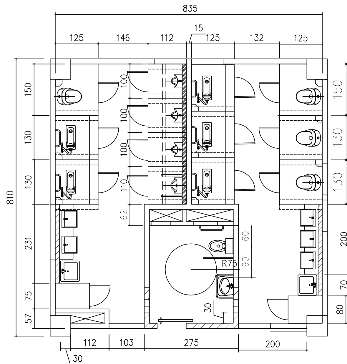
國中廁所一樓(性別友善)隔間平面圖
